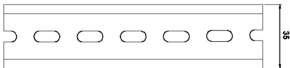
ADMISSIBLE DIN-RAIL: TS35/7.5 OR TS35/15
